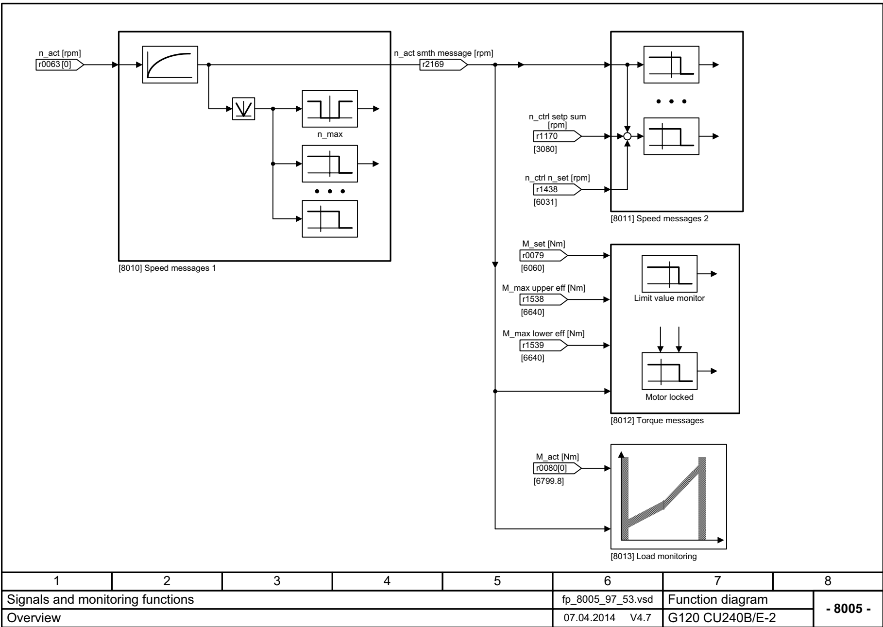
Fig. 3-135 8005 – Overview
