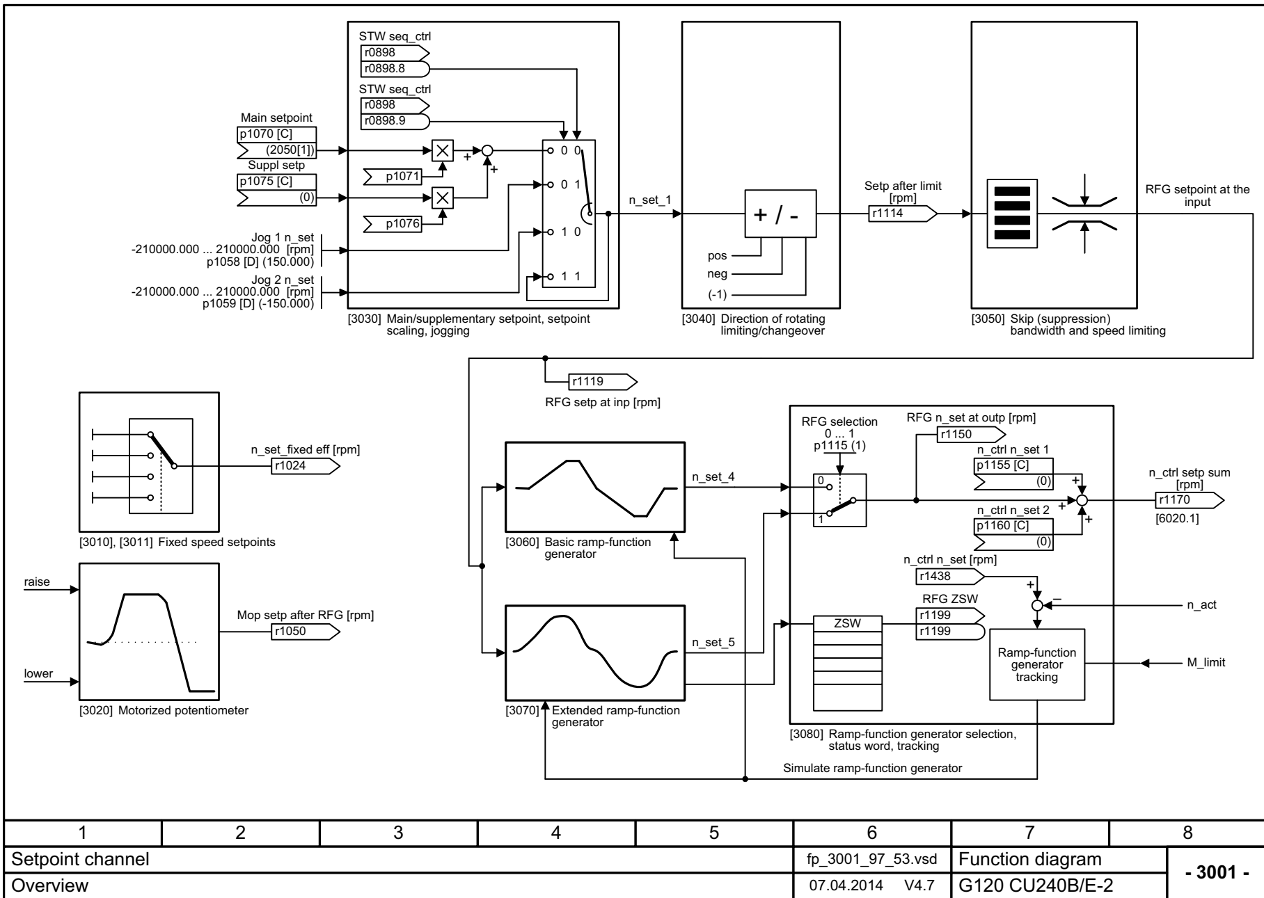
Fig. 3-75 3001 – Overview
