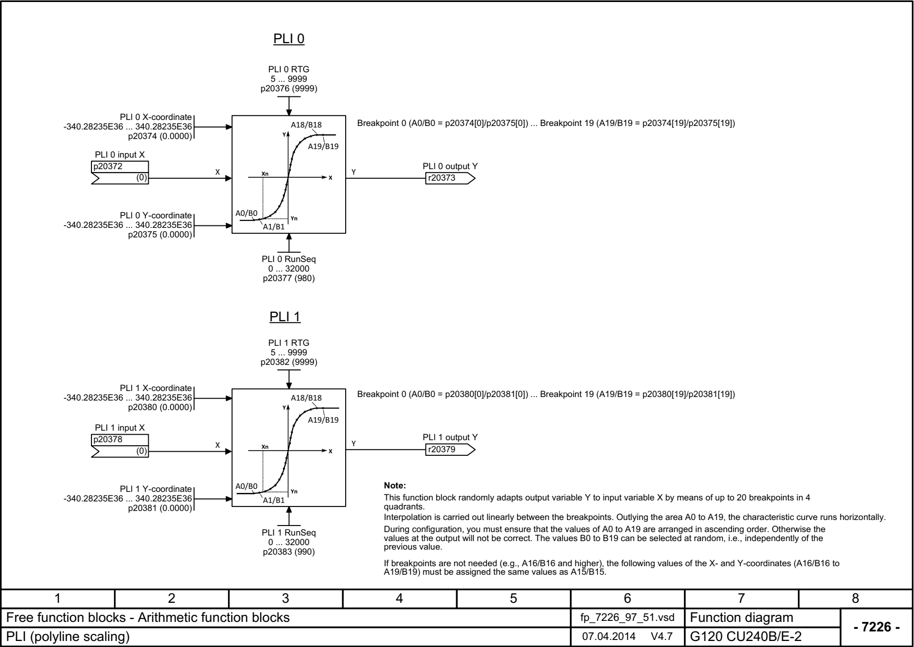
Fig. 3-120 7226 – PLI (polyline scaling)
